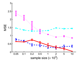
(d) Gaussian k = 8
